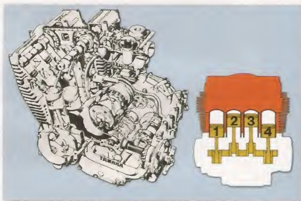
Motor policilíndrico
